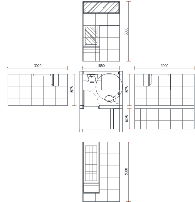
Toilet Karyawan sisi Musholla
