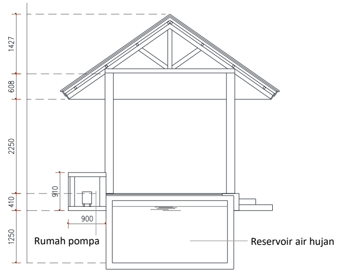
POTONGAN
