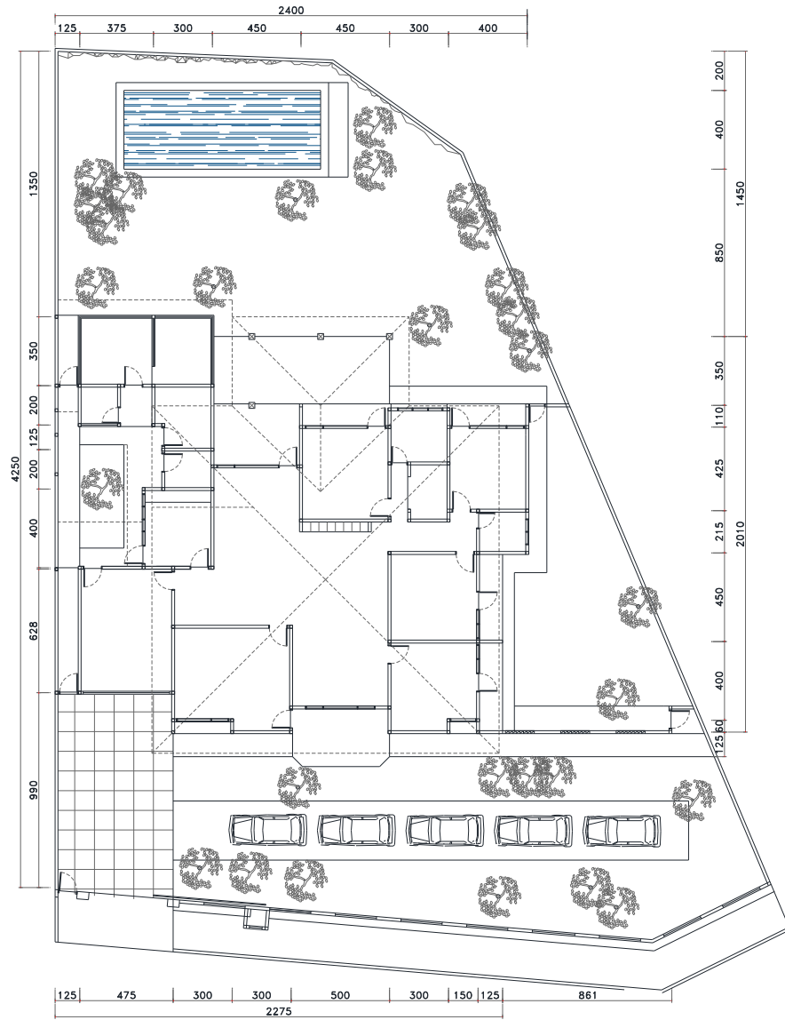
DENAH EKSTING
