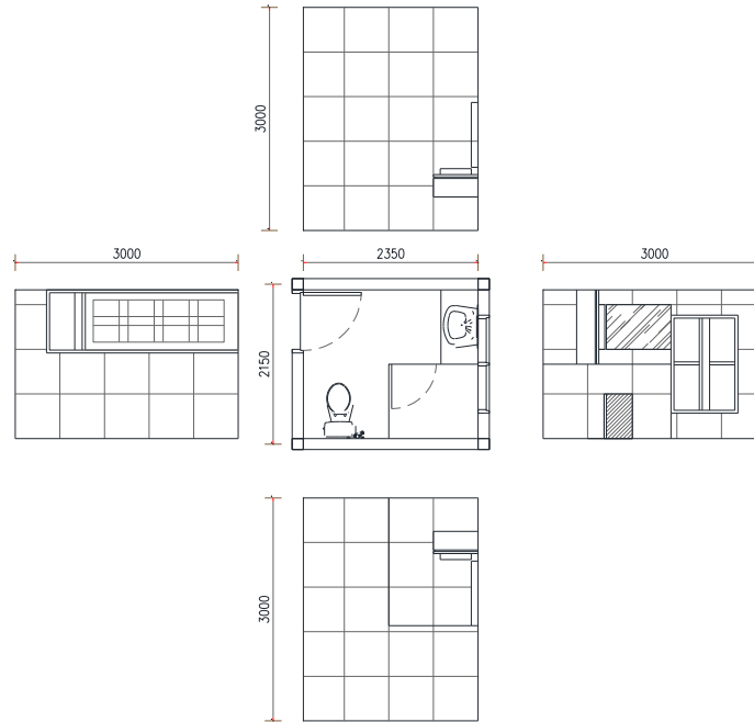
Toilet Karyawan sisi Taman samping
