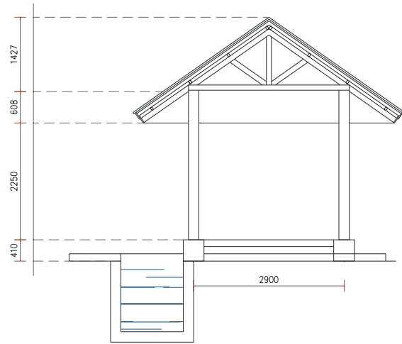
POTONGAN
