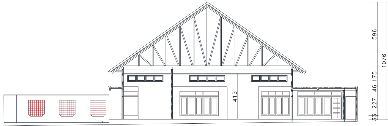
POTONGAN B-B
